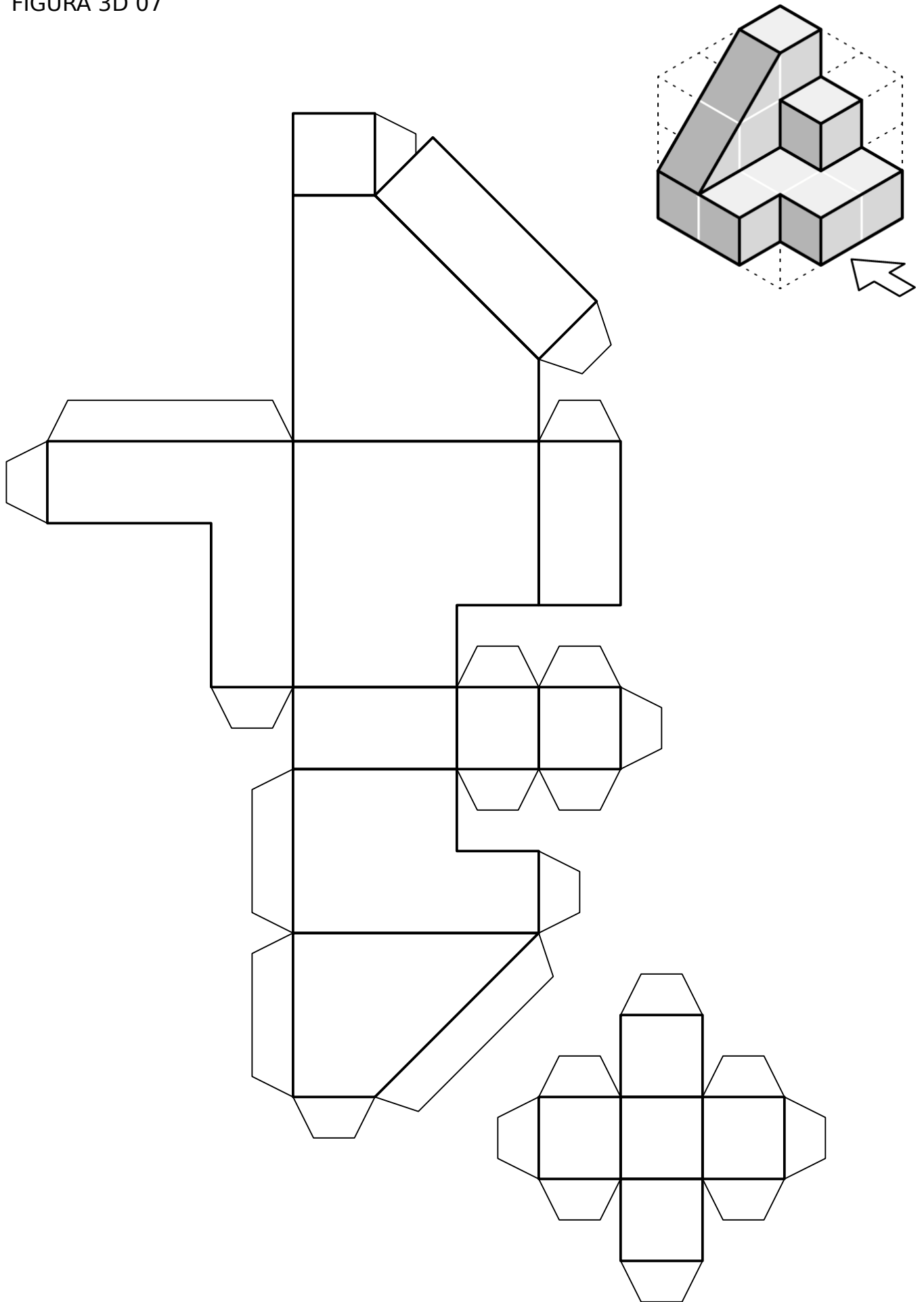
FIGURA 3D 07
